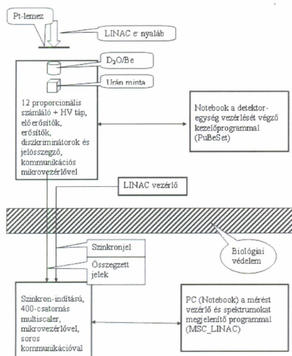
6. Ábra. Az elektronika blokkvázlata.
