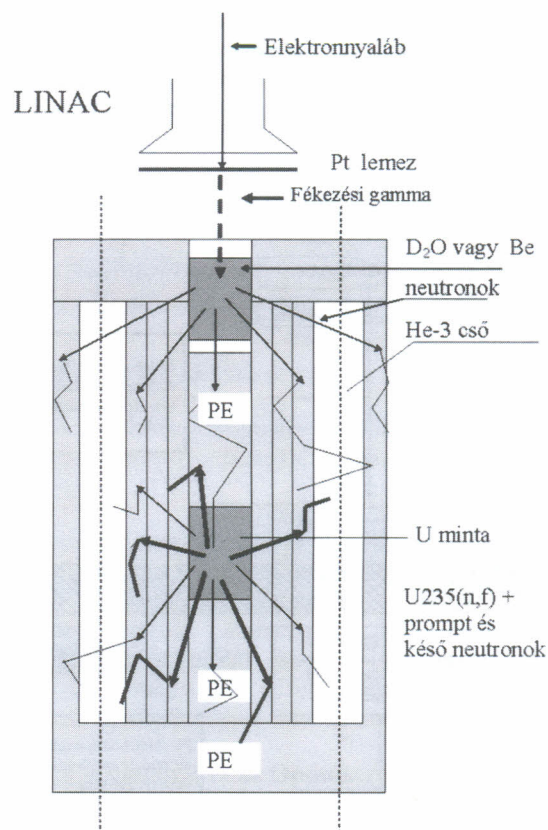
5. Ábra. A kísérleti elrendezés.
