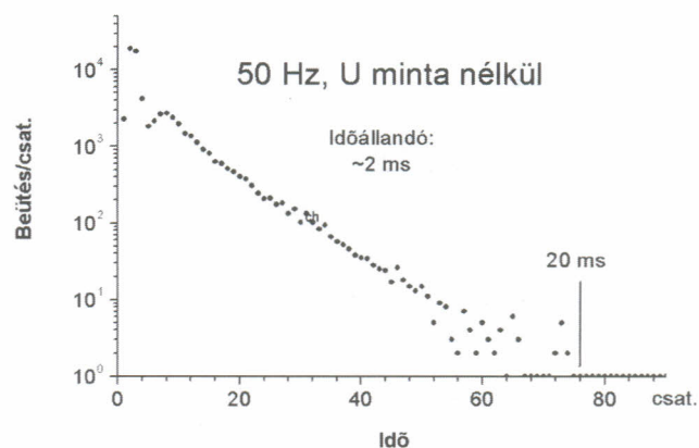
7. Ábra. Az interrogáló 50 Hz-es neutronimpulzus időspektruma Be konverterrel, U minta nélkül, 1000 besugárzási-mérési ciklus után.
